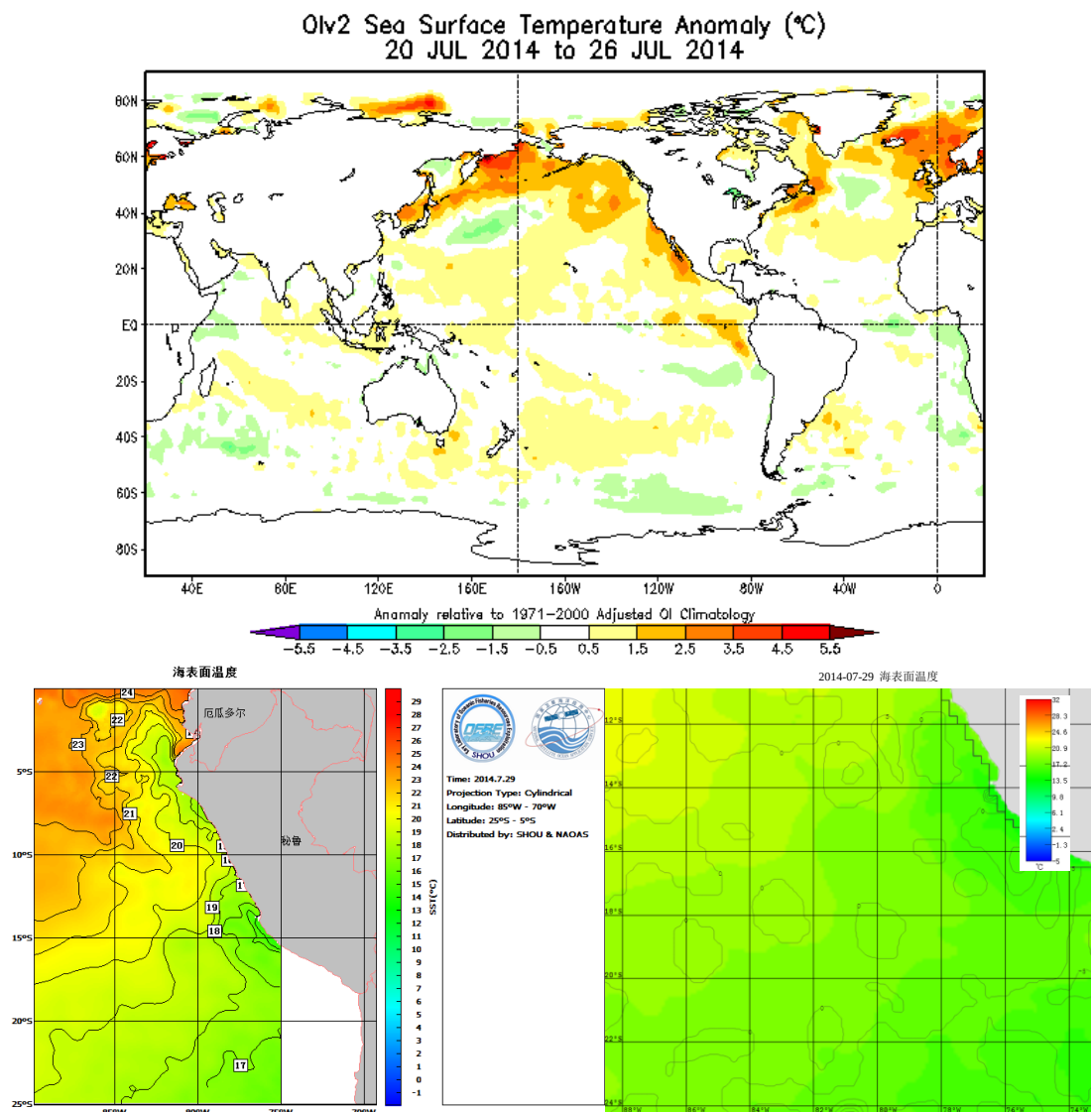
图 1 水温分布图
