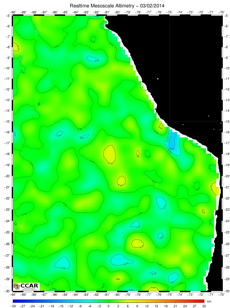
图 2 海面高度分布图
