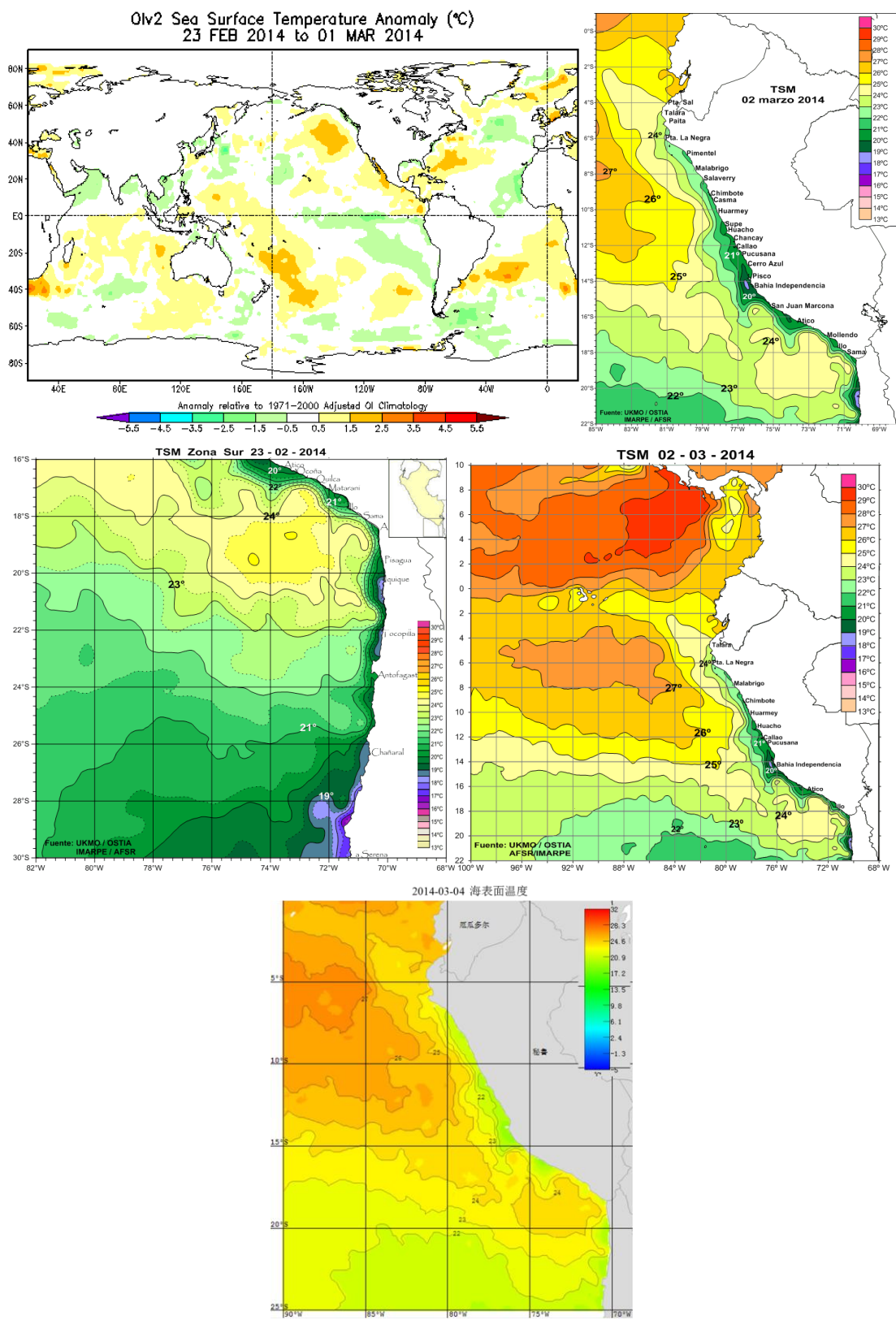
图1 水温分布图
