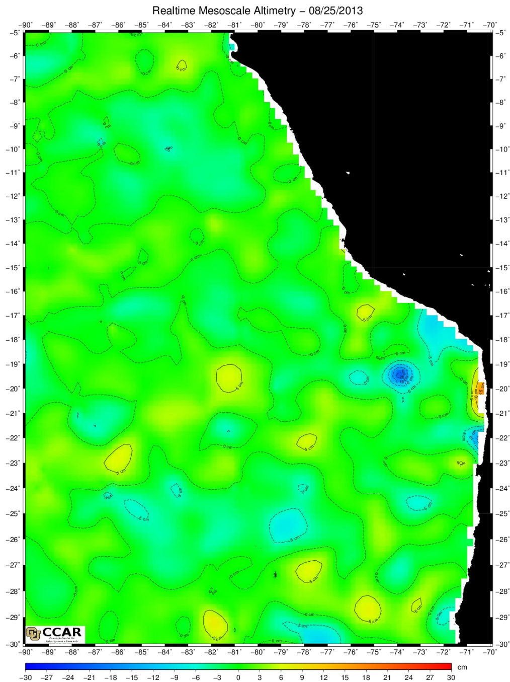
图 2 海面高度分布图
