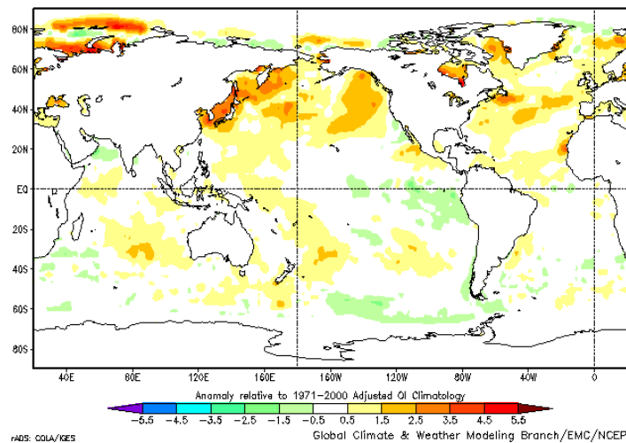
图 1 水温分布图
