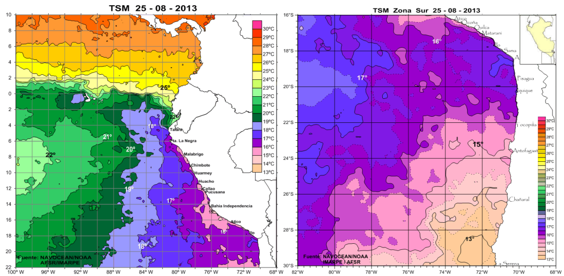
海面温度
