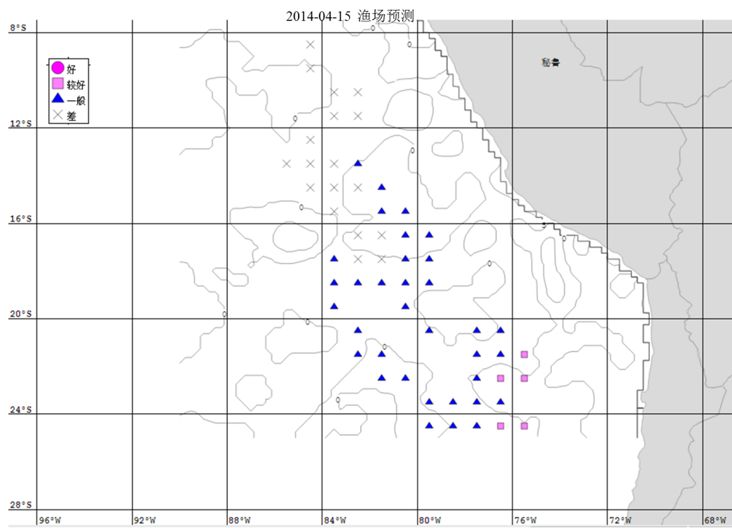
图 3 渔场预测图
