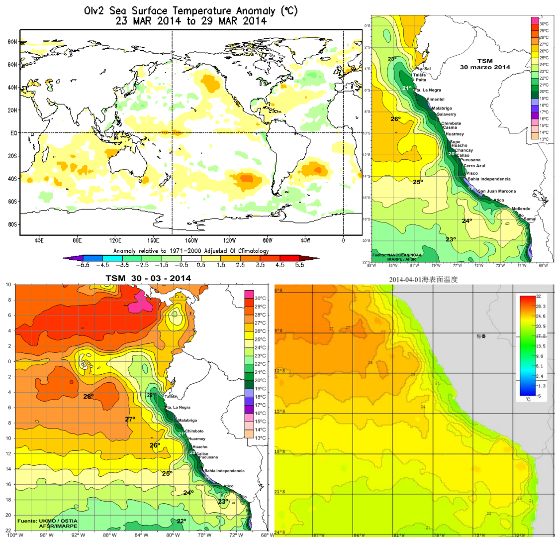
图 1 水温分布图
