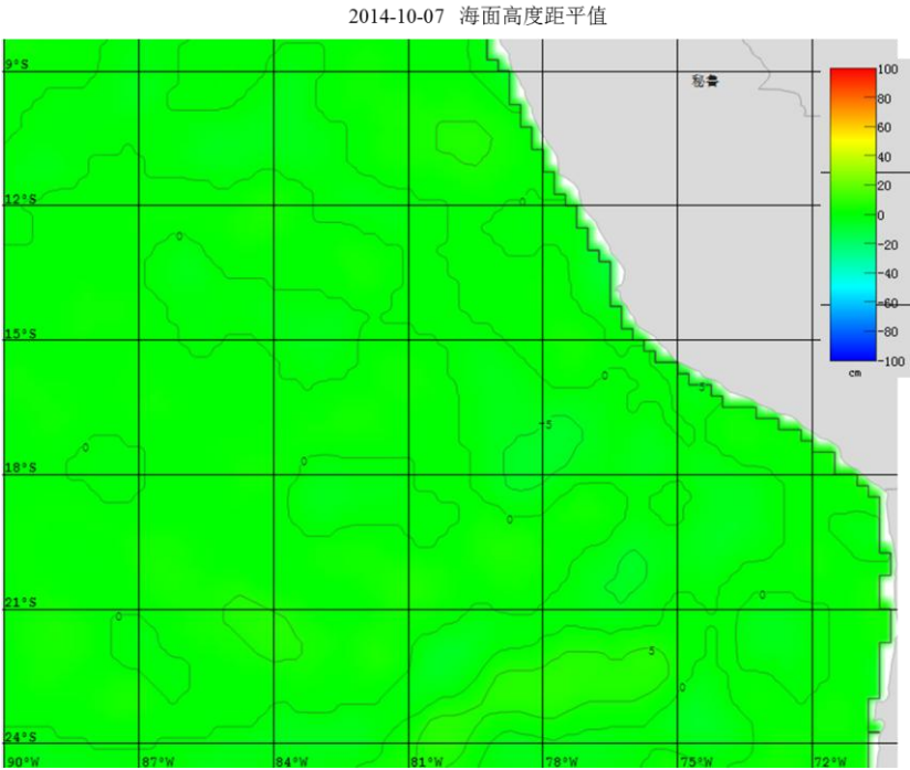
图 2 海面高度分布图
