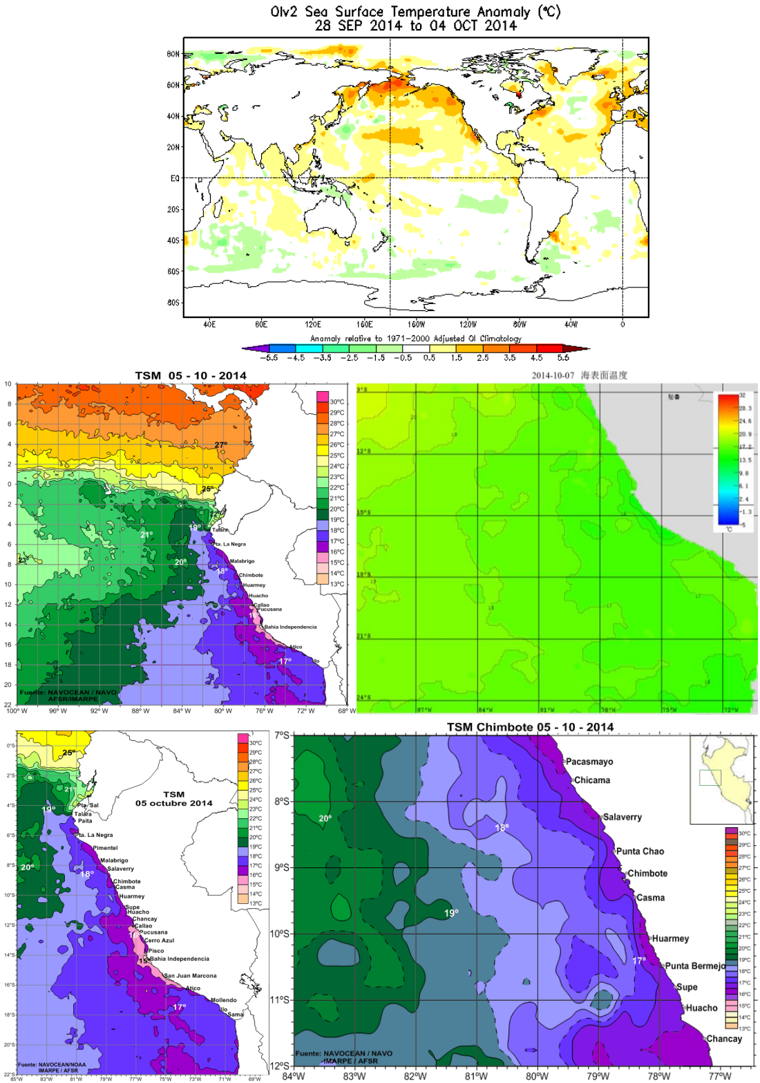
图 1 水温分布图
