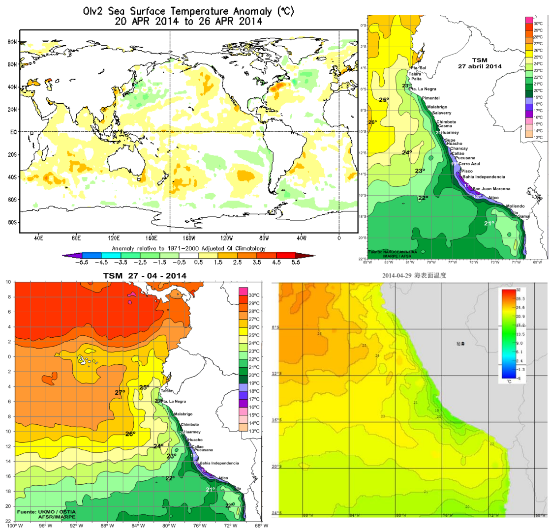
图 1 水温分布图
