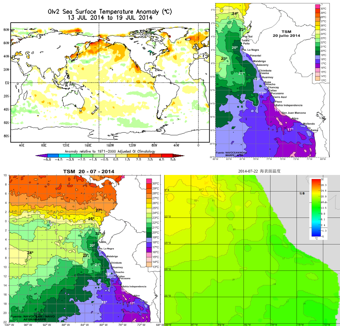
图 1 水温分布图
