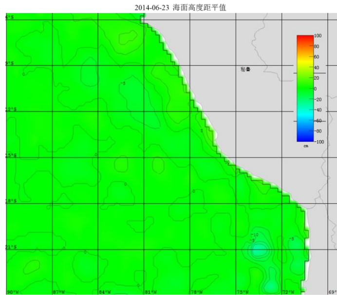
图 2 海面高度分布图
