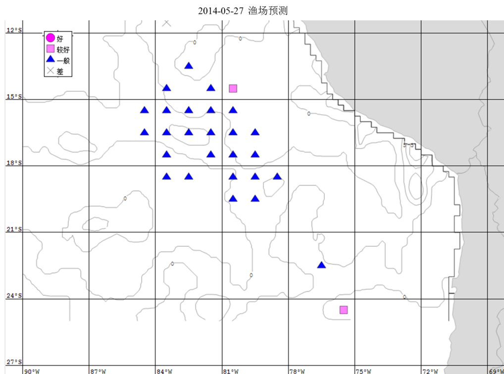
图 3 渔场预测图
