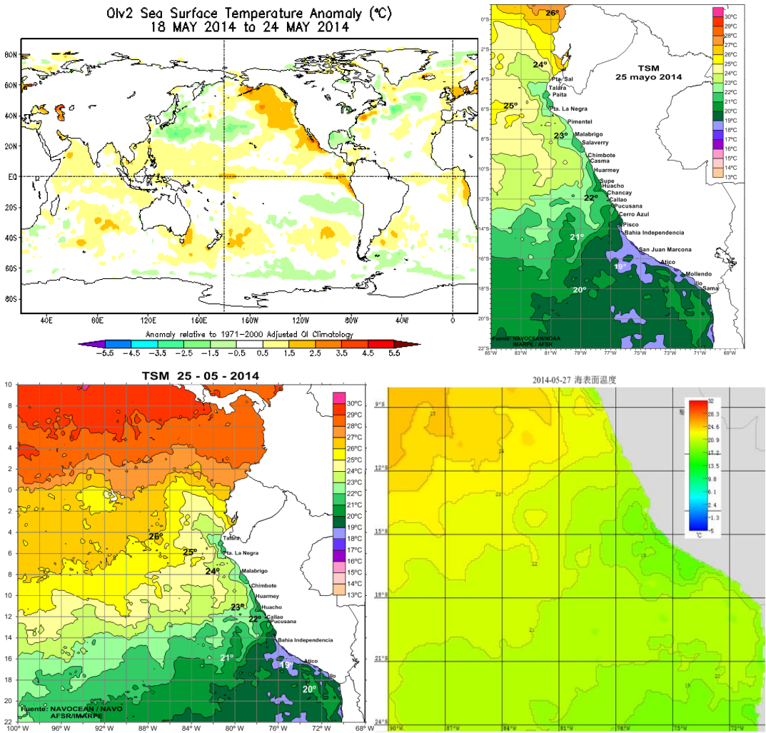
图 1 水温分布图
