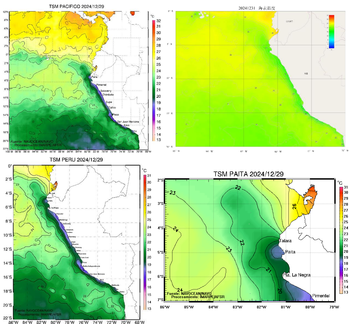
图 1 水温分布图
