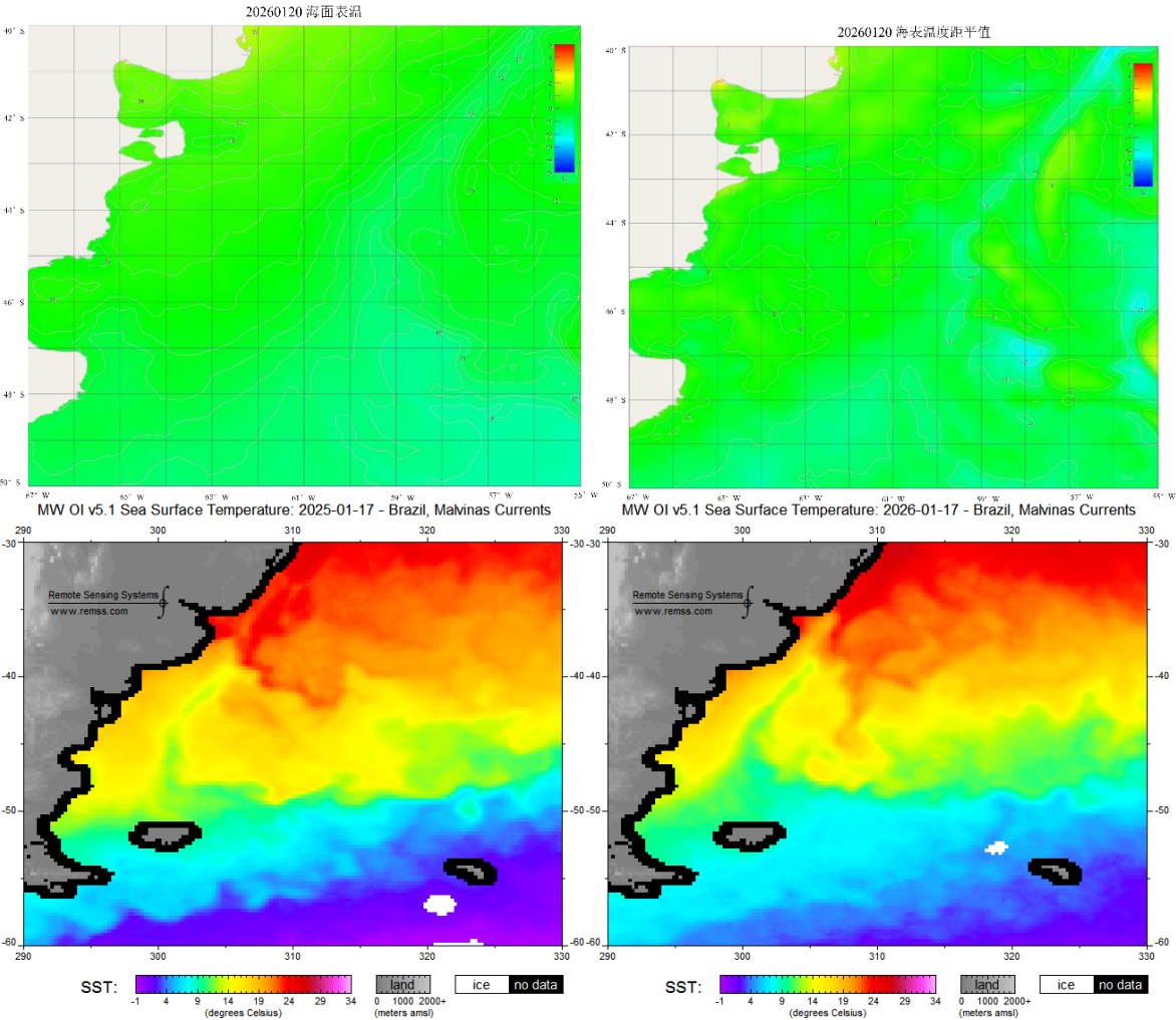
图 1 表温分布图
