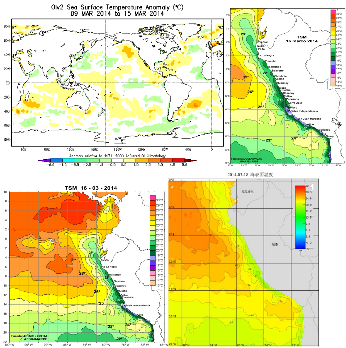
图 1 水温分布图
